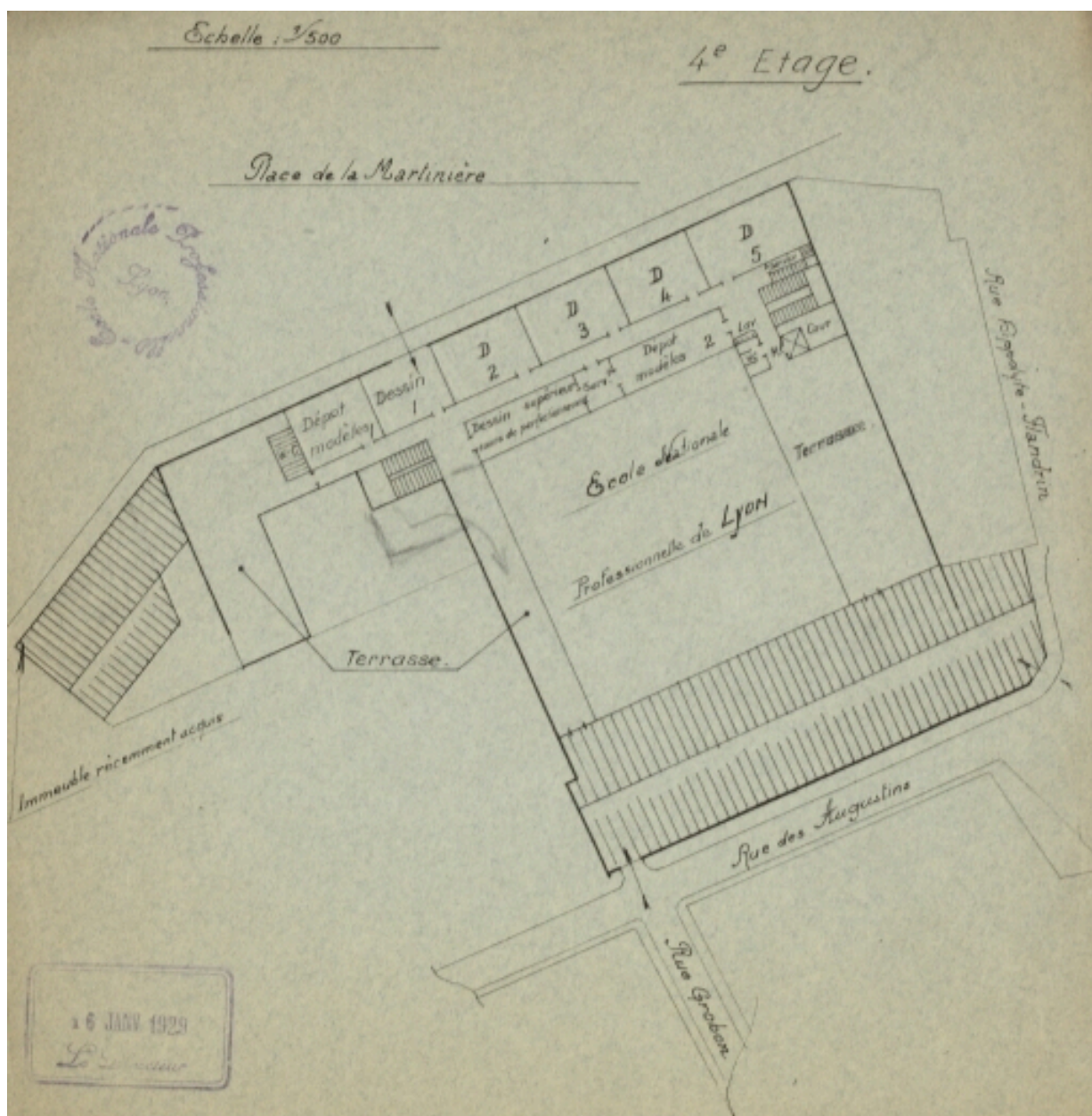
Plans de la Martinière garçons, 16 janvier 1929, 1/500e. 4e étage. Document figuré. 16 janvier 1929. 1:500. Archives de la Fondation Martin. non coté
