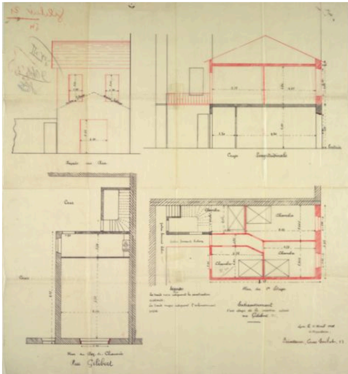
Plan de la maison occupant la partie sud de la parcelle, 1906
