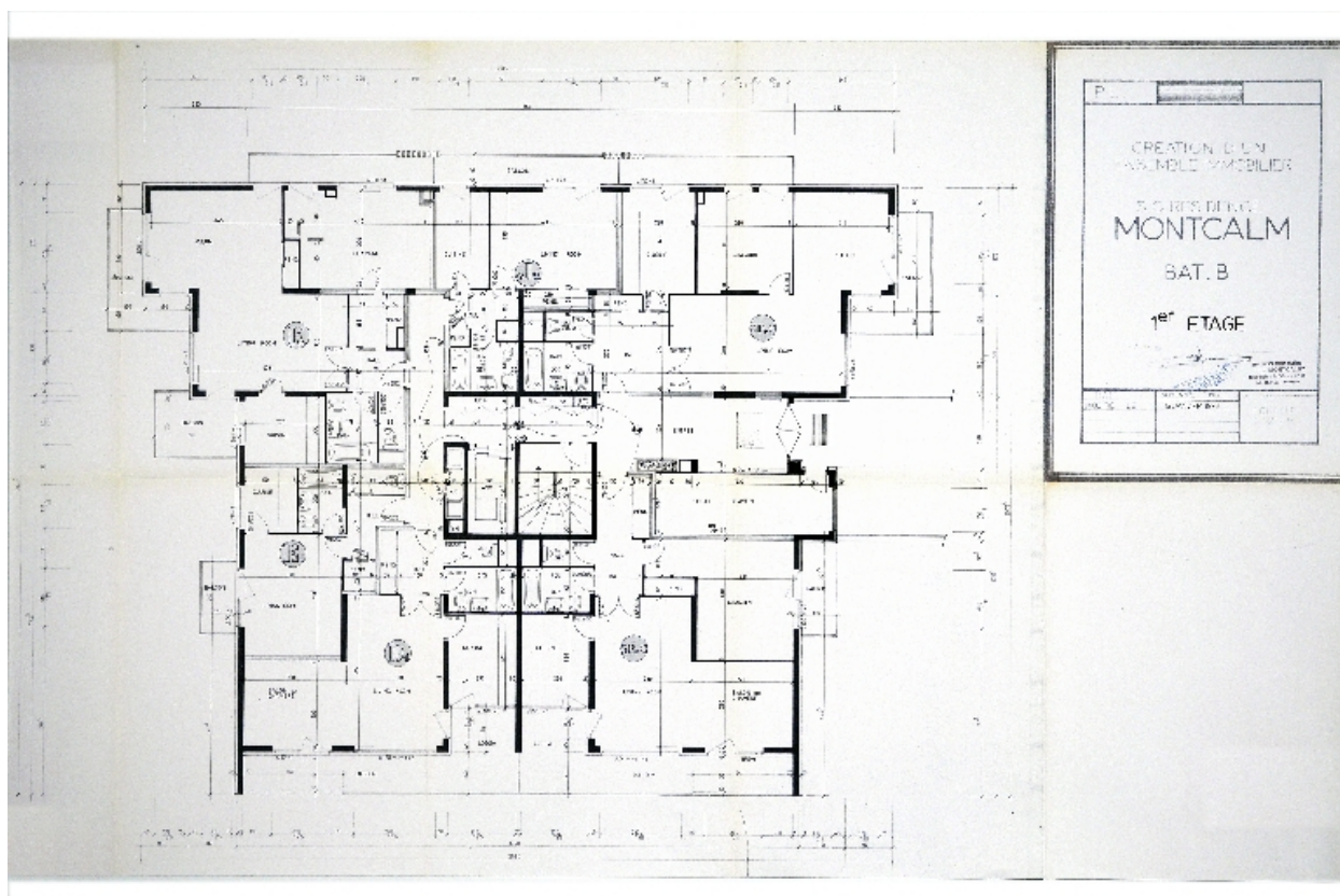
Bât. B : Plan du 1er étage
