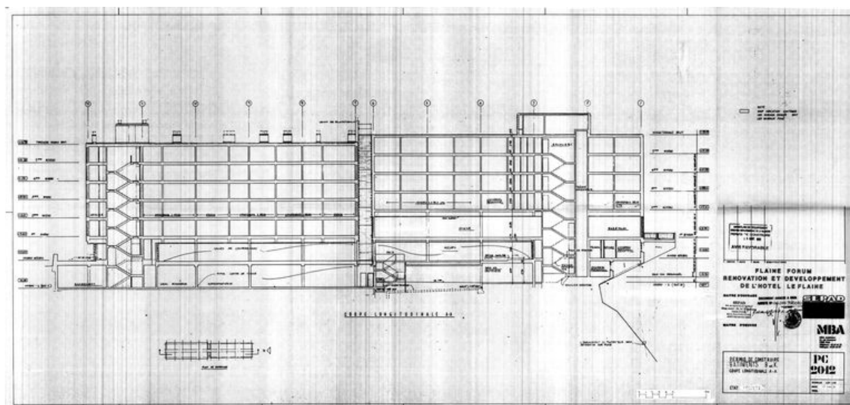
Rénovation et développement de l'hôtel le Flaine. Bâtiments B et K. Coupe longitudinale A-A. Etat projeté. MBA maître d'oeuvre, 10 mai 1991 (AC Arâches-la-Frasse)
