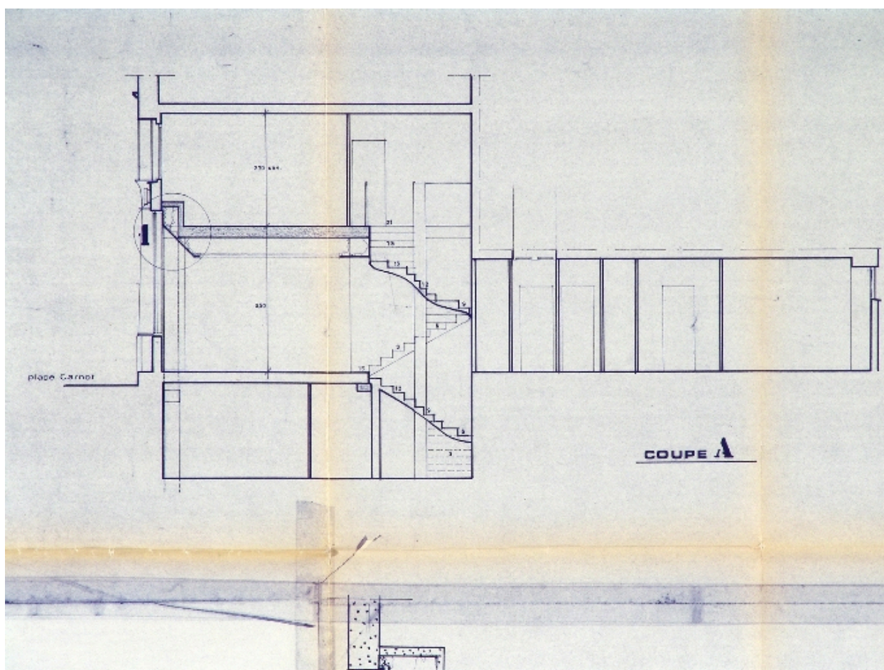
Coupe A
