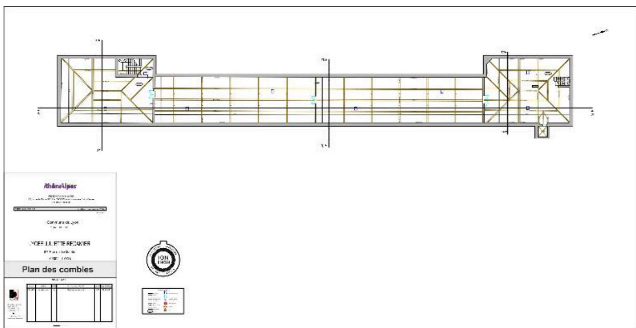
Plan des combles. Dess. AGATHE, 2012
