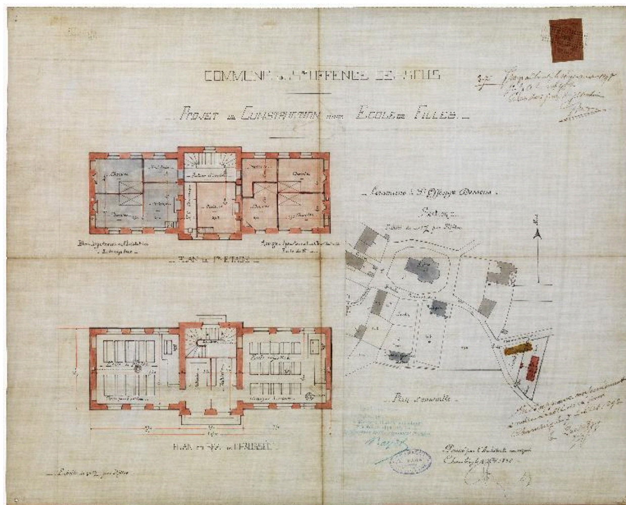
Projet de construction d'une école de filles, plan du rez-de-chaussée, 1er étage. Faga, 1896.
