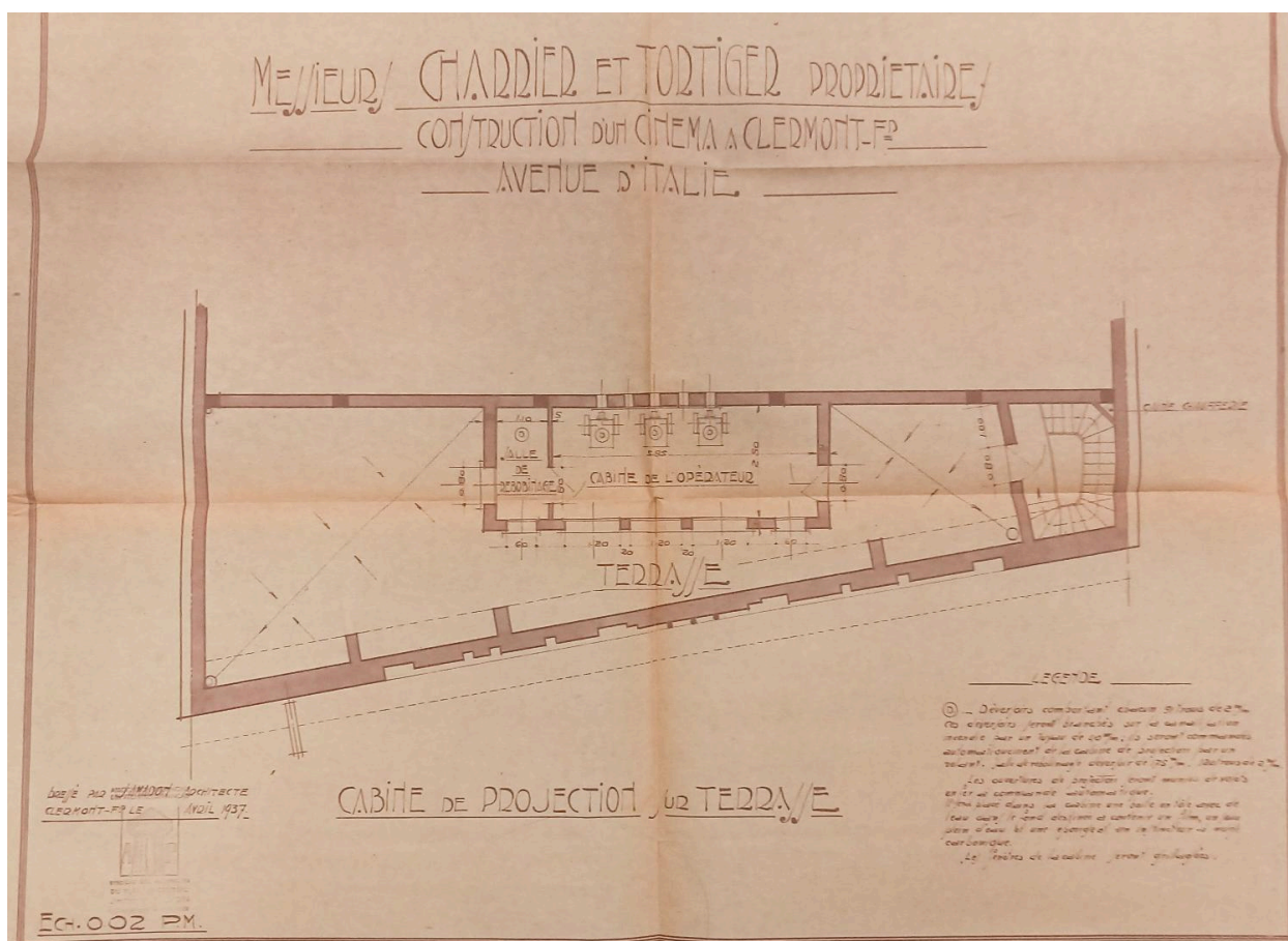
Plan de la cabine de projection sur la terrasse, cinéma le Vox
