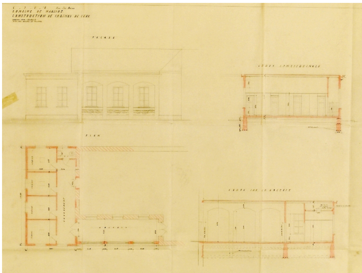
Cabines de luxe : plan, coupes et élévations, 1951
