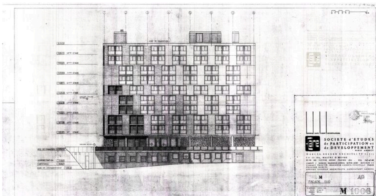
Hôtel M. Elévation sud. Marcel Breuer architecte, 27 janvier 1971 (AC Arâches-la Frasse)
