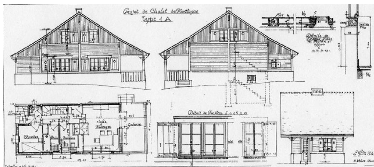
Plan, élévations et détails du chalet de type 1A : Stéphane Weber, 4 juin 1926
