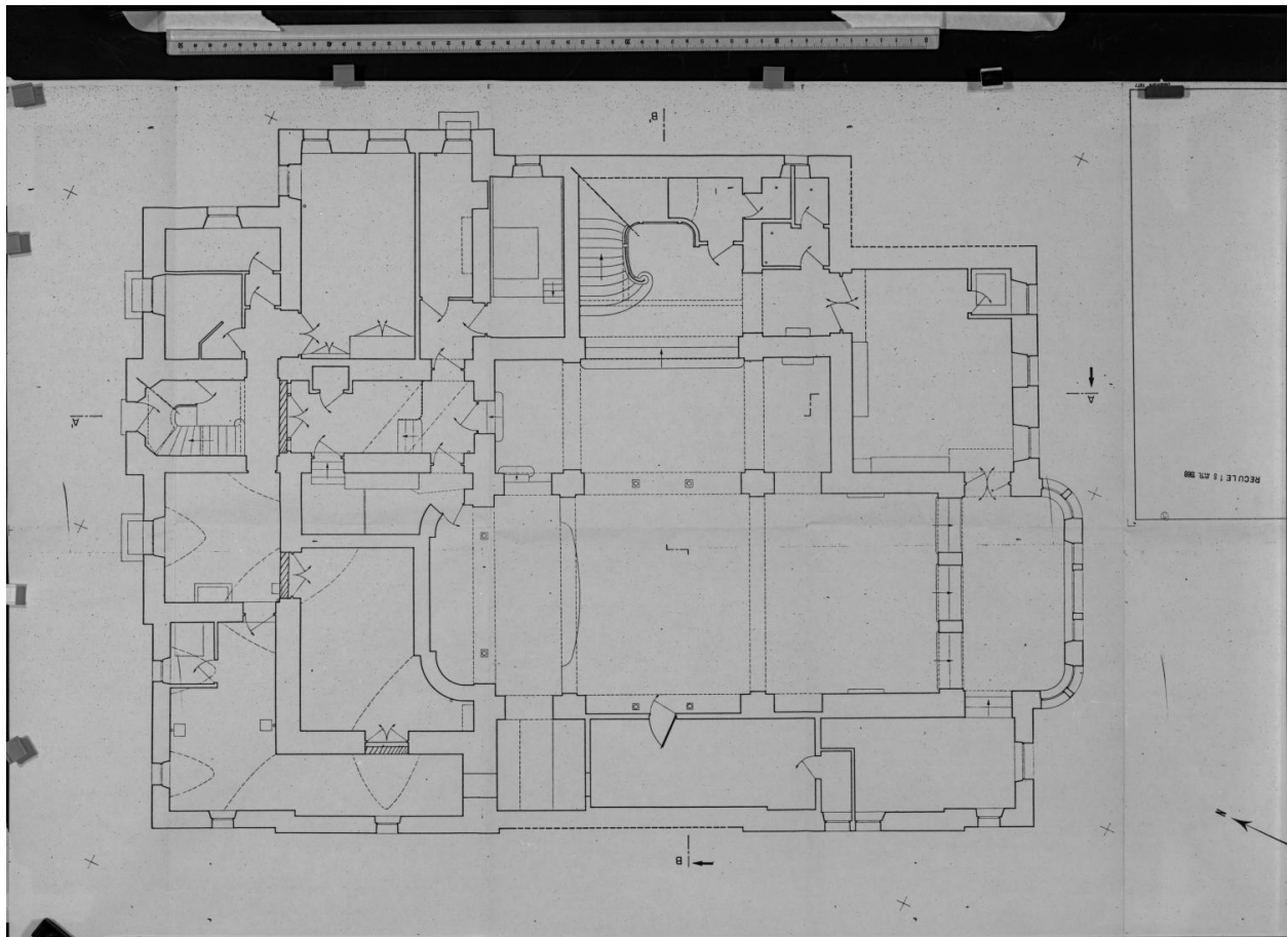
Plan des sous-sol
