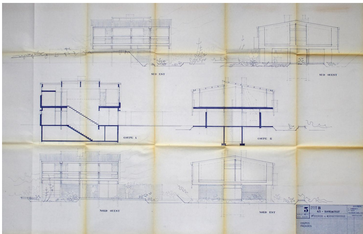
Romagnat, la maison B., façades et coupes, Lucien Ambrosetti et J.-P. Gauer architectes, juin 1969 (archives municipales de Romagnat).
