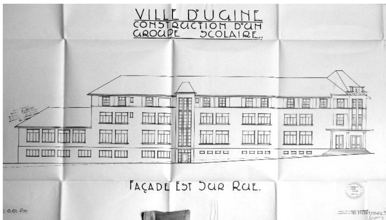
Ville d'Ugine, Construction d'un groupe scolaire. Façade est sur rue, Projet, A. Bugnard Novembre 1931 (AD Savoie, 2 O 2966)
