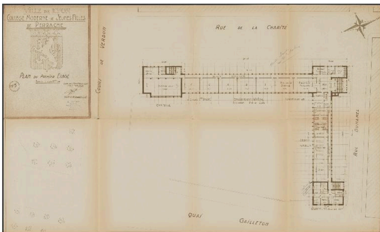
Plan du 1er étage, par E. Payen, 1954 (AC Lyon, 838 WP 001)
