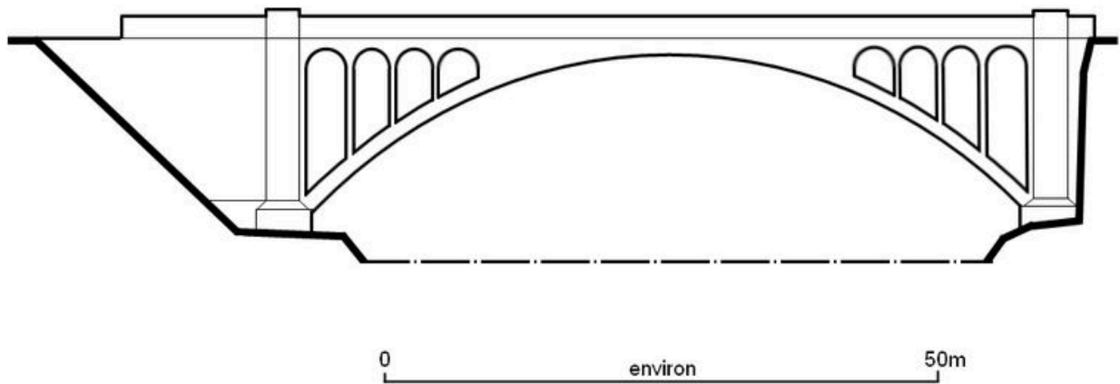
Elévation aval (relevé schématique)
