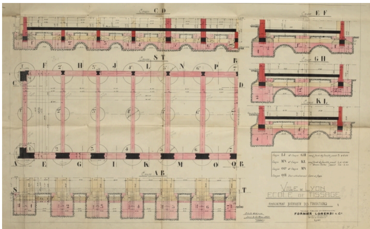
Ecole de tissage, plan des fondations. 7 février 1929. Fornier Lorensi & Cie, ingénieurs constructeurs. (AC Lyon. 511 WP 002)
