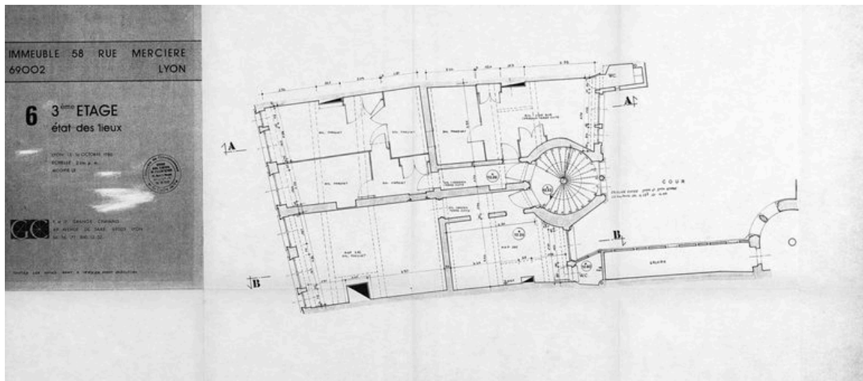
Plan du 3e étage, état des lieux. 1980 CRMH Rhône-Alpes. 1 | 11 MHAA-99-463
