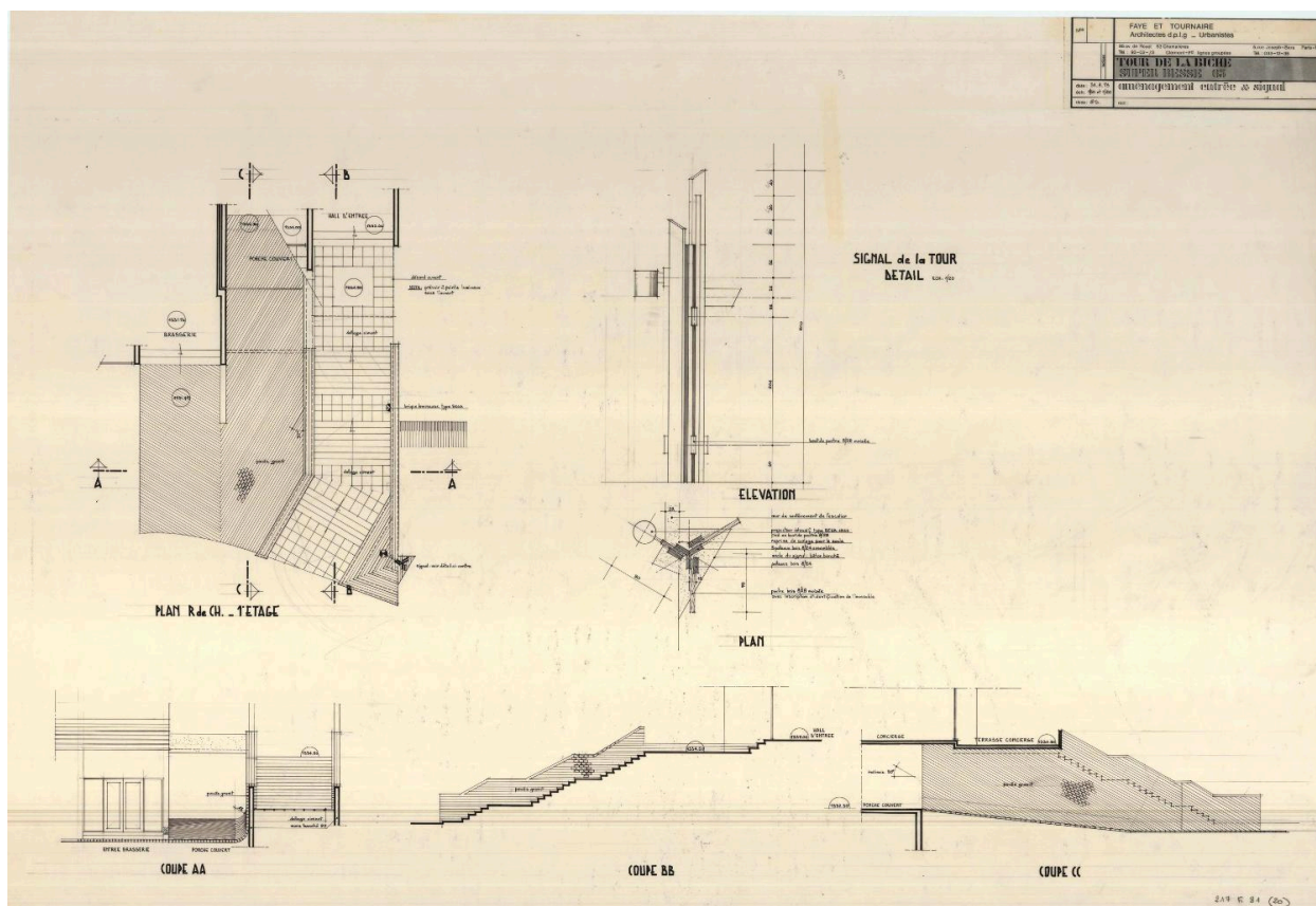
Super-Besse, la Tour de la Biche, plan d'aménagement de l'entrée principale et du signal prévu à côté de l'entrée, août 1973, Faye et Tournaire architectes (AD63, 217 Fi 81 / 20).
