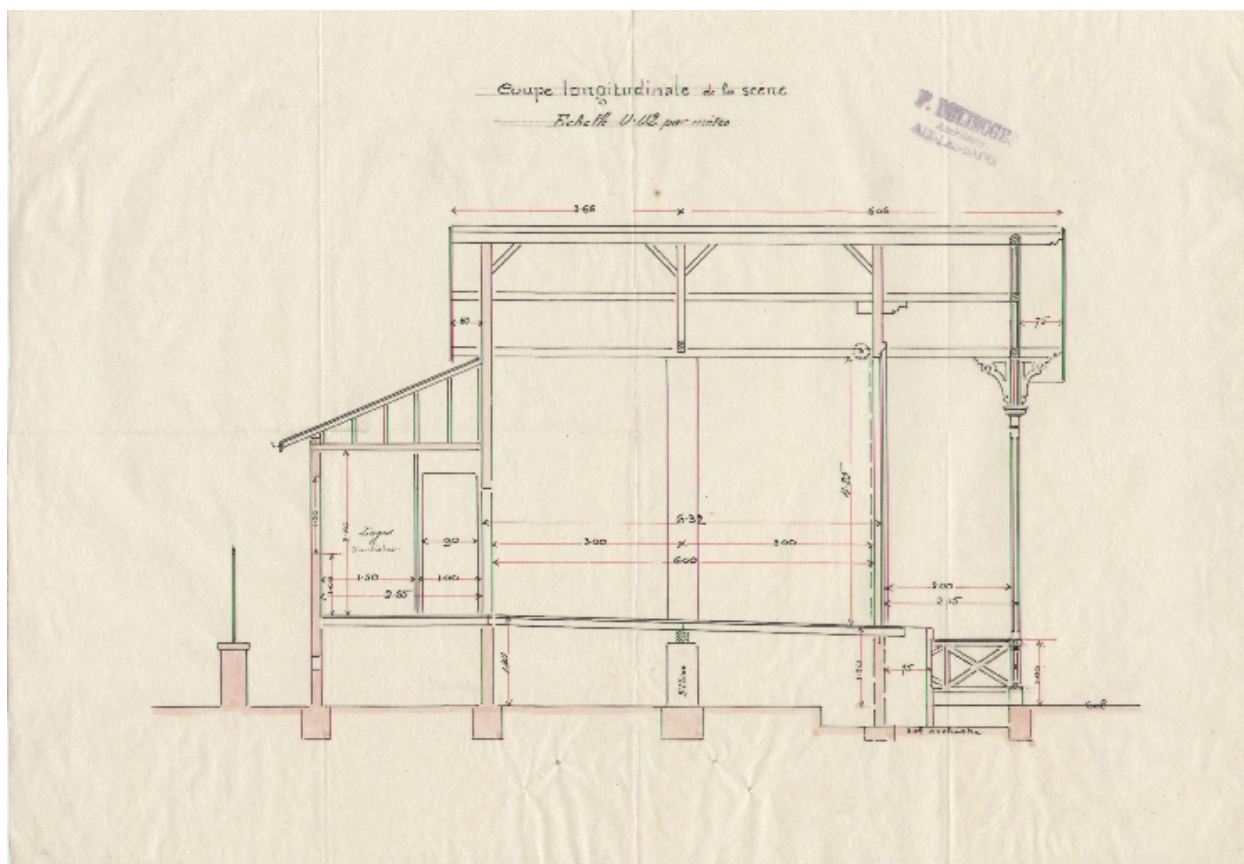
Coupe de la scène du théâtre
