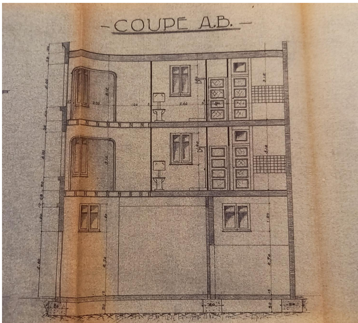
Coupe (projet non réalisé 1954)
