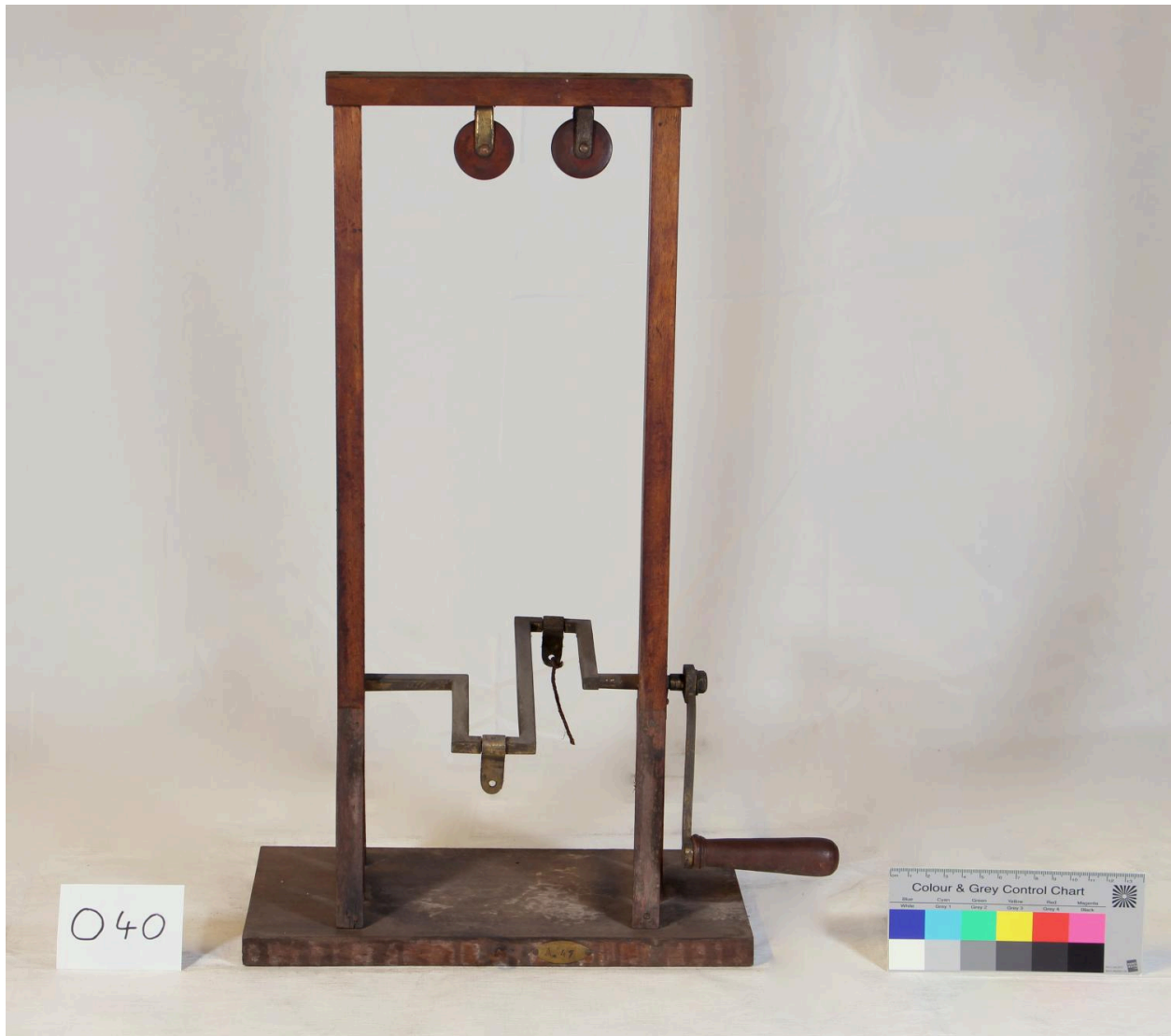
Transformation de mouvement (liste supplémentaire n°040)
