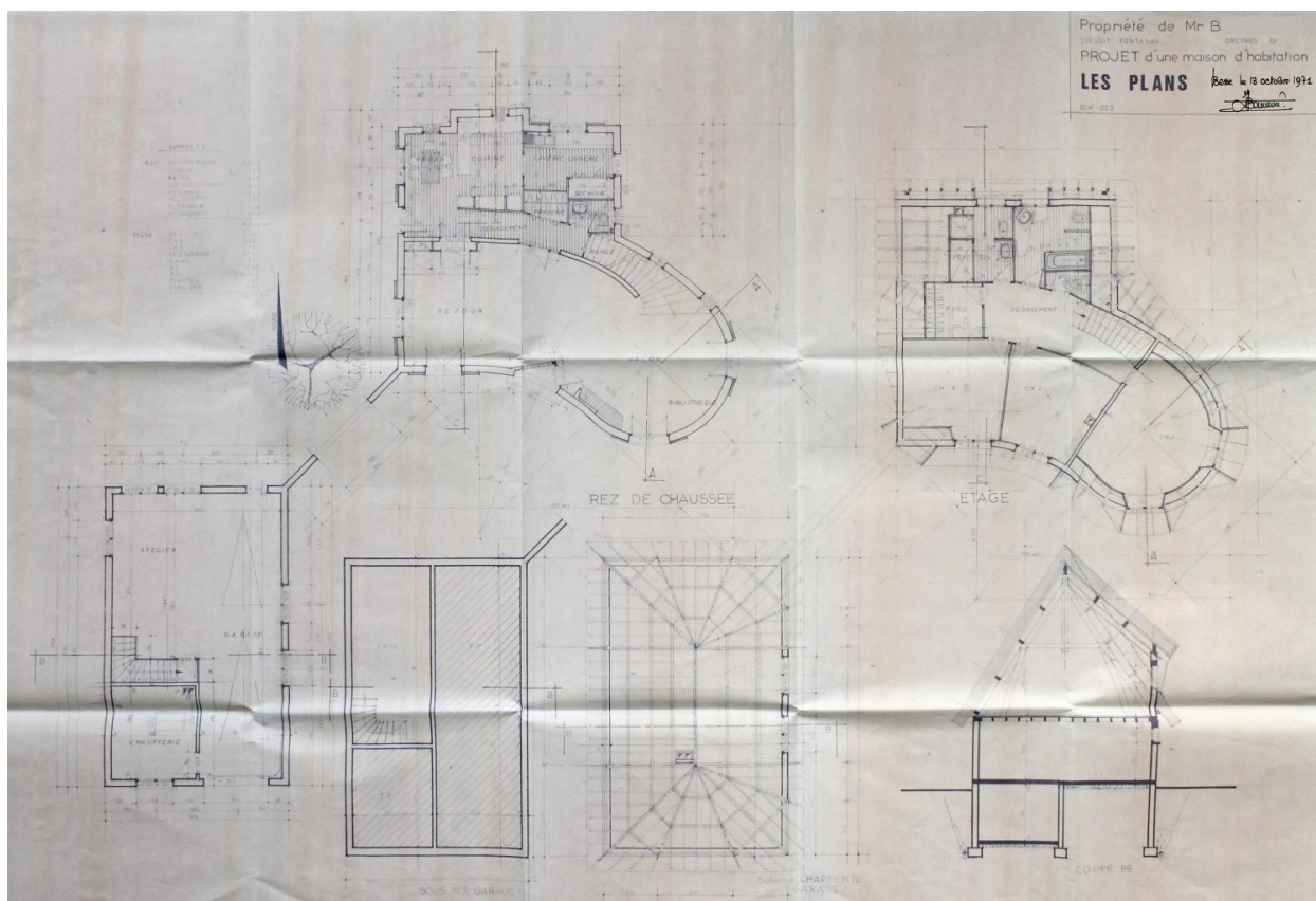
Orcines, la maison Bo., plans du rez-de-chaussée, de l'étage et du garage, schéma de charpente et coupes, anonyme, 1971 (archives municipales d'Orcines).
