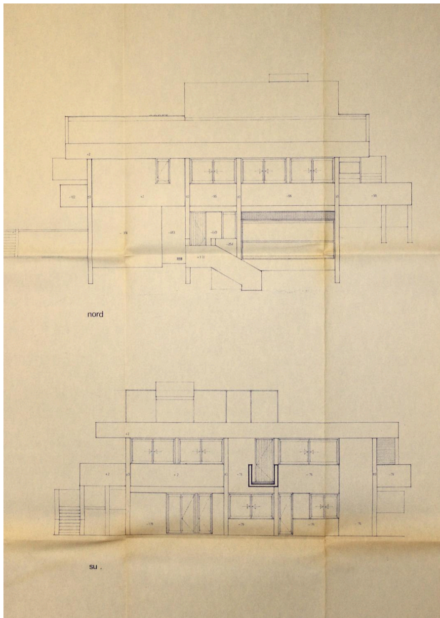
Clermont-Ferrand, la villa F., façades nord et sud, Michel Vigneron architecte, septembre 1970 - mars 1971 (archives municipales de Clermont-Ferrand).
