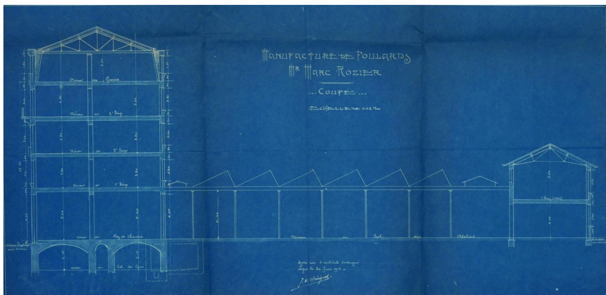
Coupe de l'usine Rozier, 1913 (AC Lyon : 314W512- dossier 471 )
