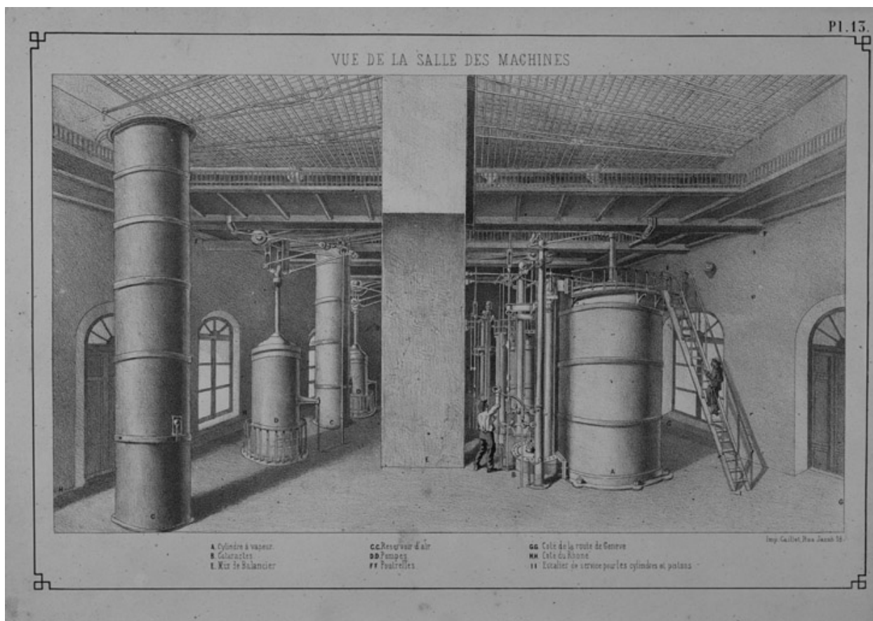
Vue de la salle des machines
