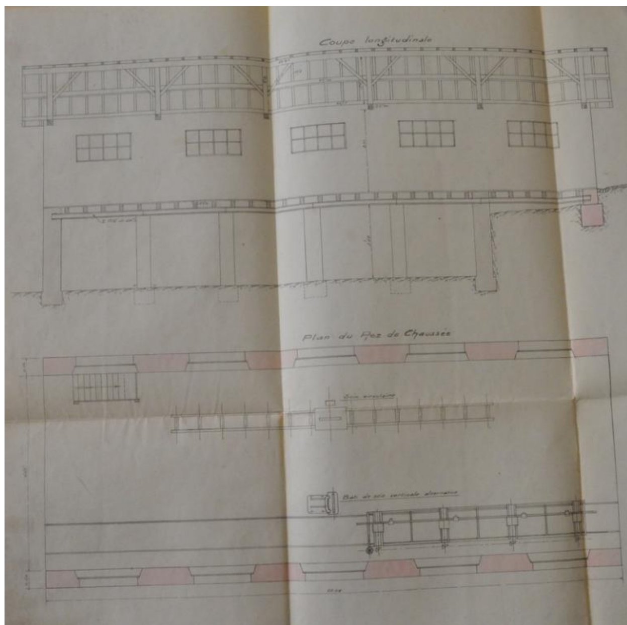
Plan de la nouvelle scierie, 1937 (FR.AD073, 201977).
