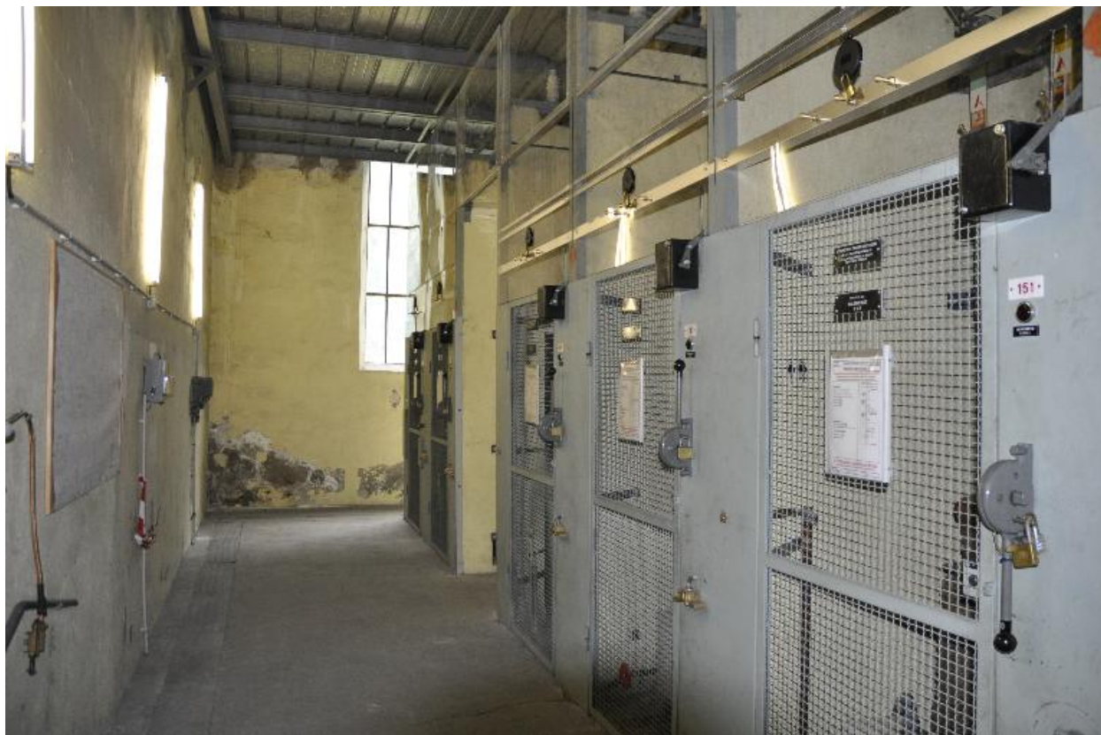
Vue des armoires des transformateurs
