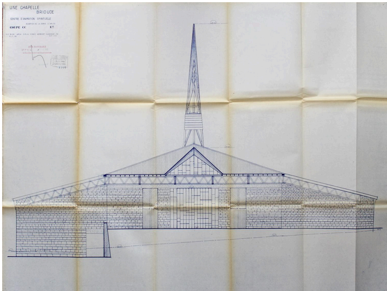
Brioude, chapelle de la Borie Darles, coupe CC sur le porche (projet non définitif), 30 mars 1965, Guy Bion architecte, Archives de la paroisse Saint-Julien de Brioude.
