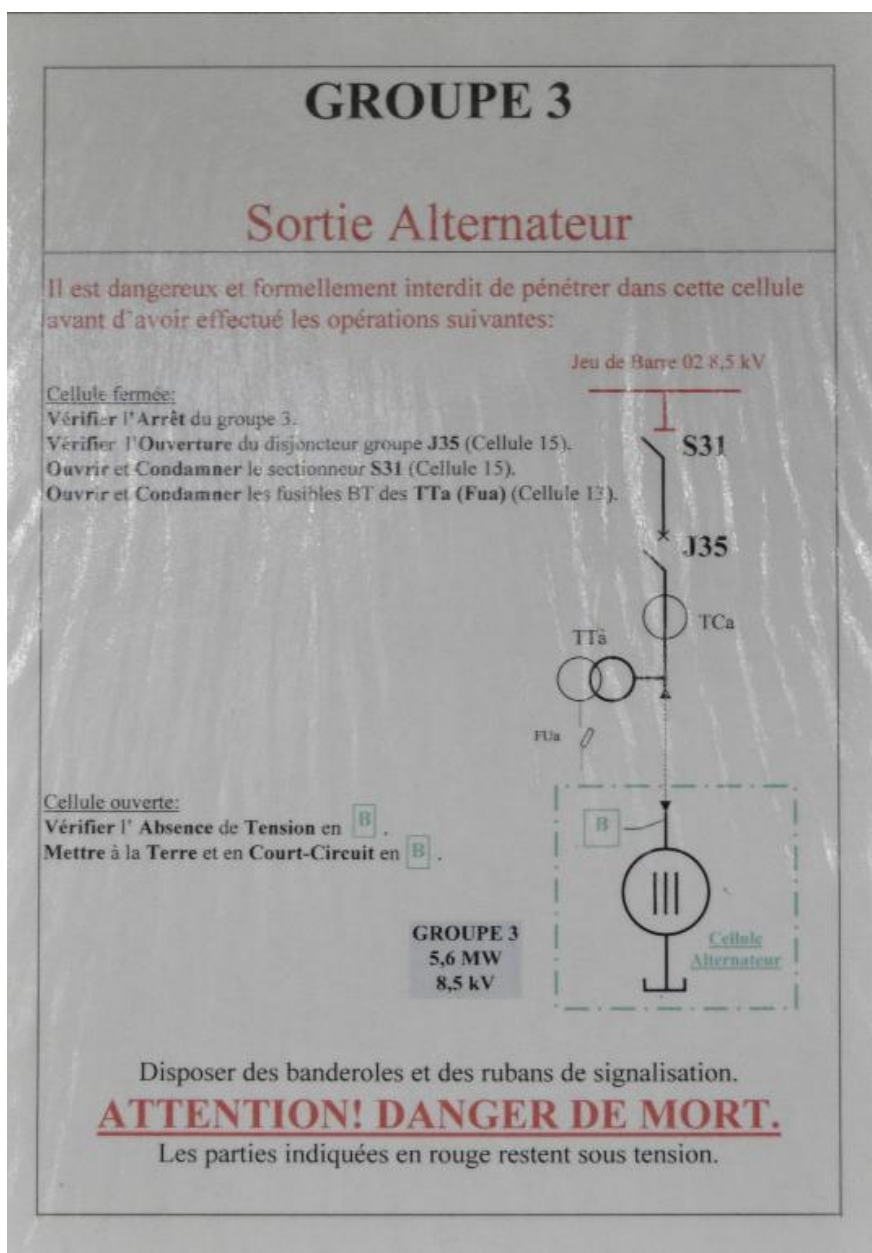
Détail de la sortie d'alternateur du groupe 3
