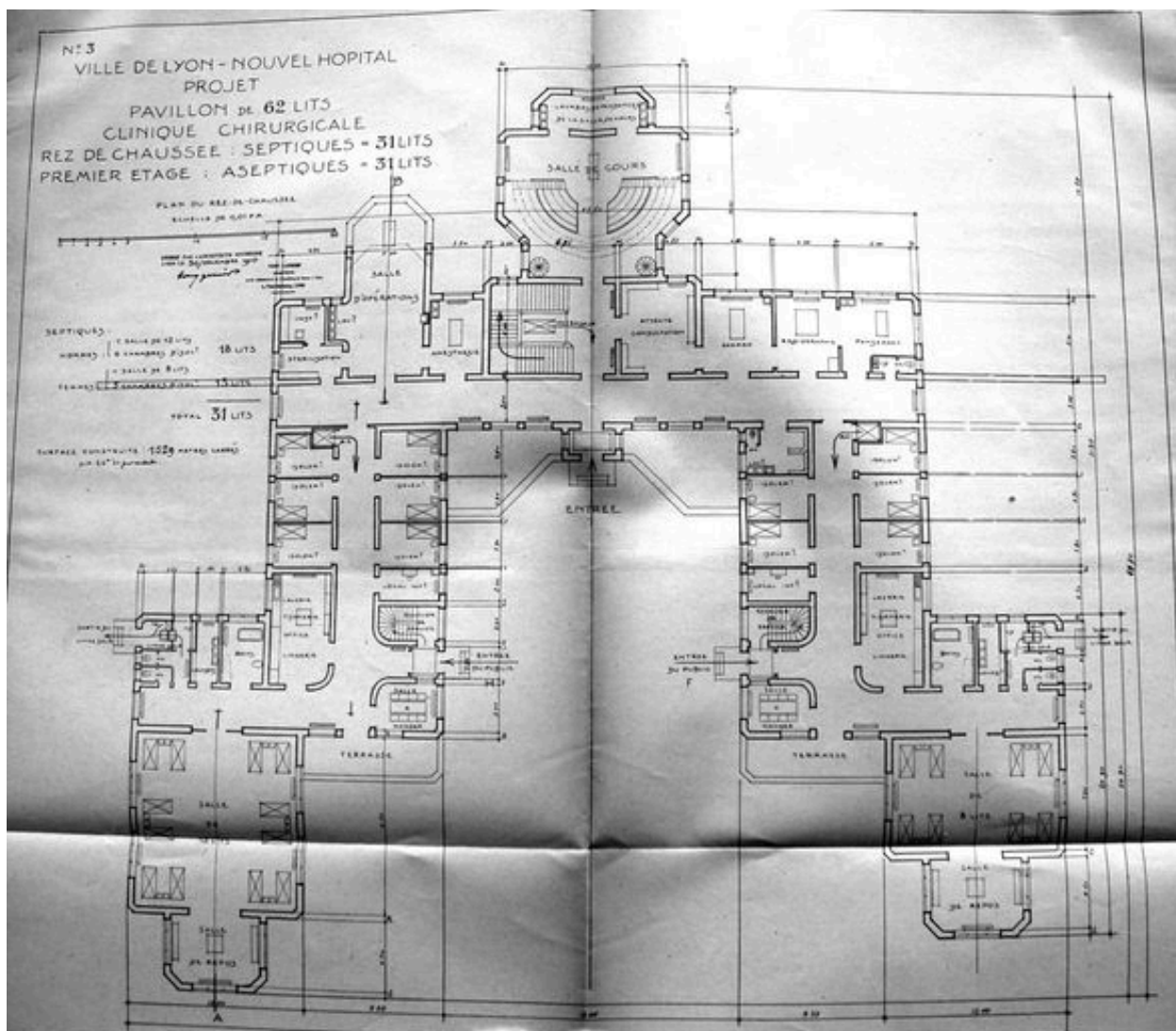
Projet. Pavillon de 62 lits. Clinique chirurgicale. Plan du rez-de-chaussée / Tony Garnier, 30 décembre 1910 (Arch. mun. Lyon. 959 WP 139)
