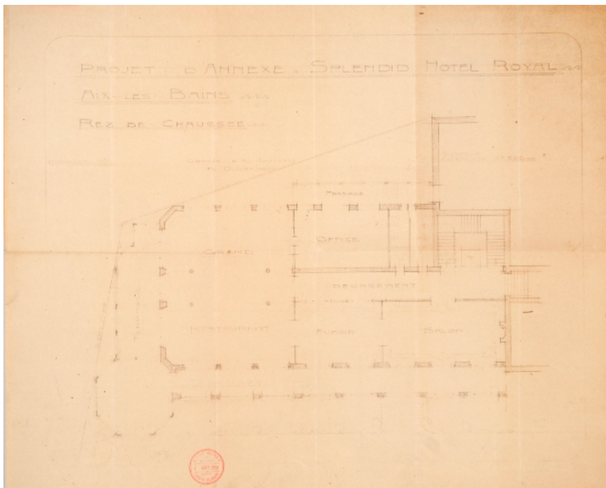
Projet du rez-de-chaussée
