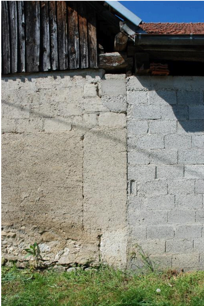
Les Farniers. Ferme, parcelle 2013 E1 84, détail de matériaux au niveau du mur pignon est
