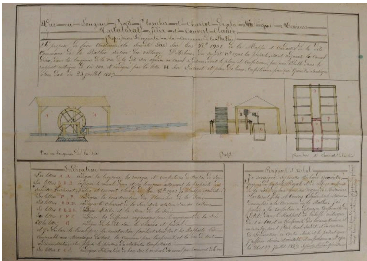
Plan du projet de scierie de Claude Convert, 1863 (FR.AD073, 82S5).
