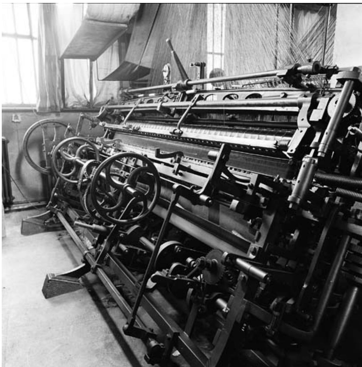
Métier à tisser la dentelle de marque Husbands classé Monument historique (Angleterre)
