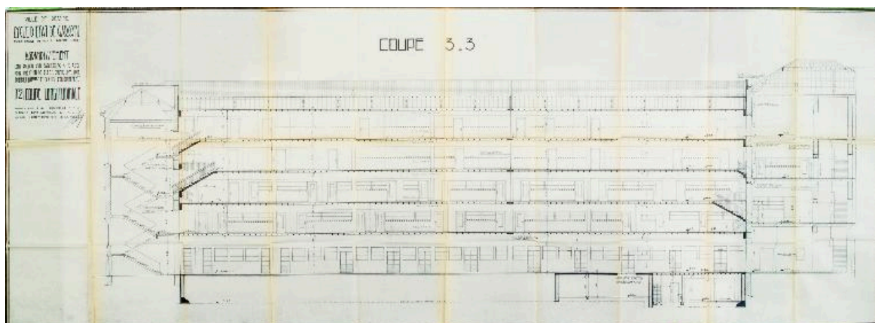
Extension du lycée. 12 : Coupe longitudinale (1963)
