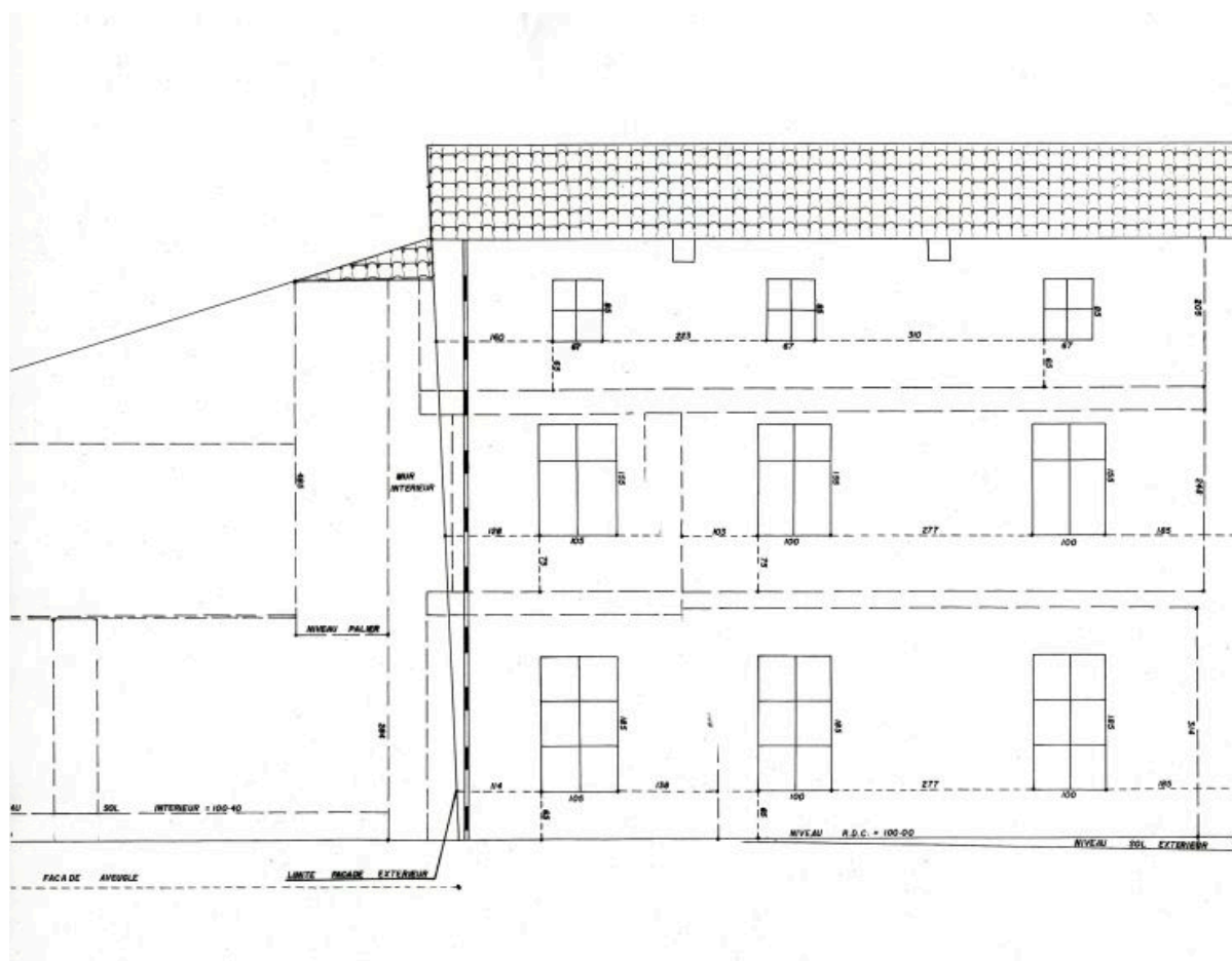
Elévation de la façade sud.
