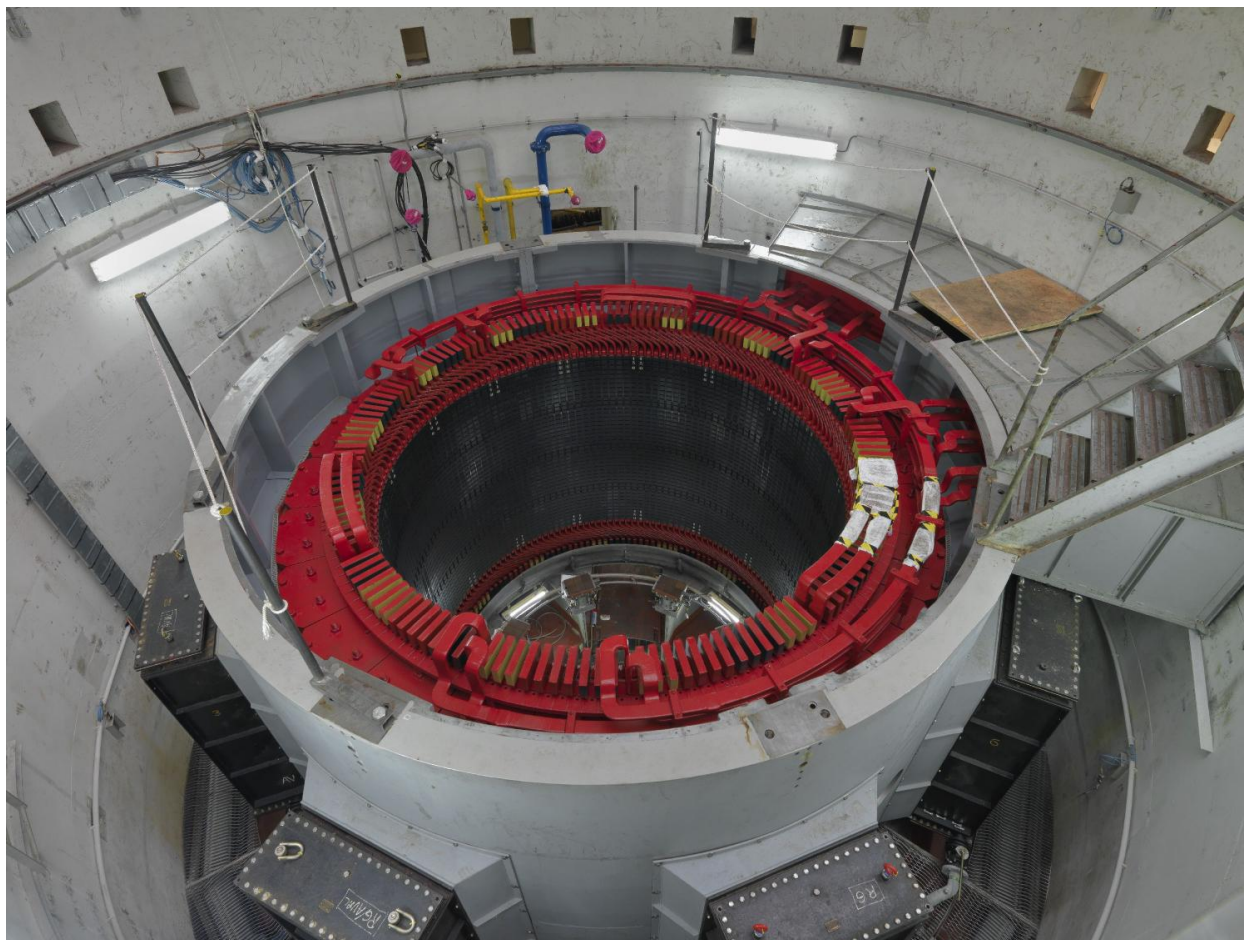
Groupe 6 en cours de rénovation, vue sur le stator rebobiné de l'alternateur
