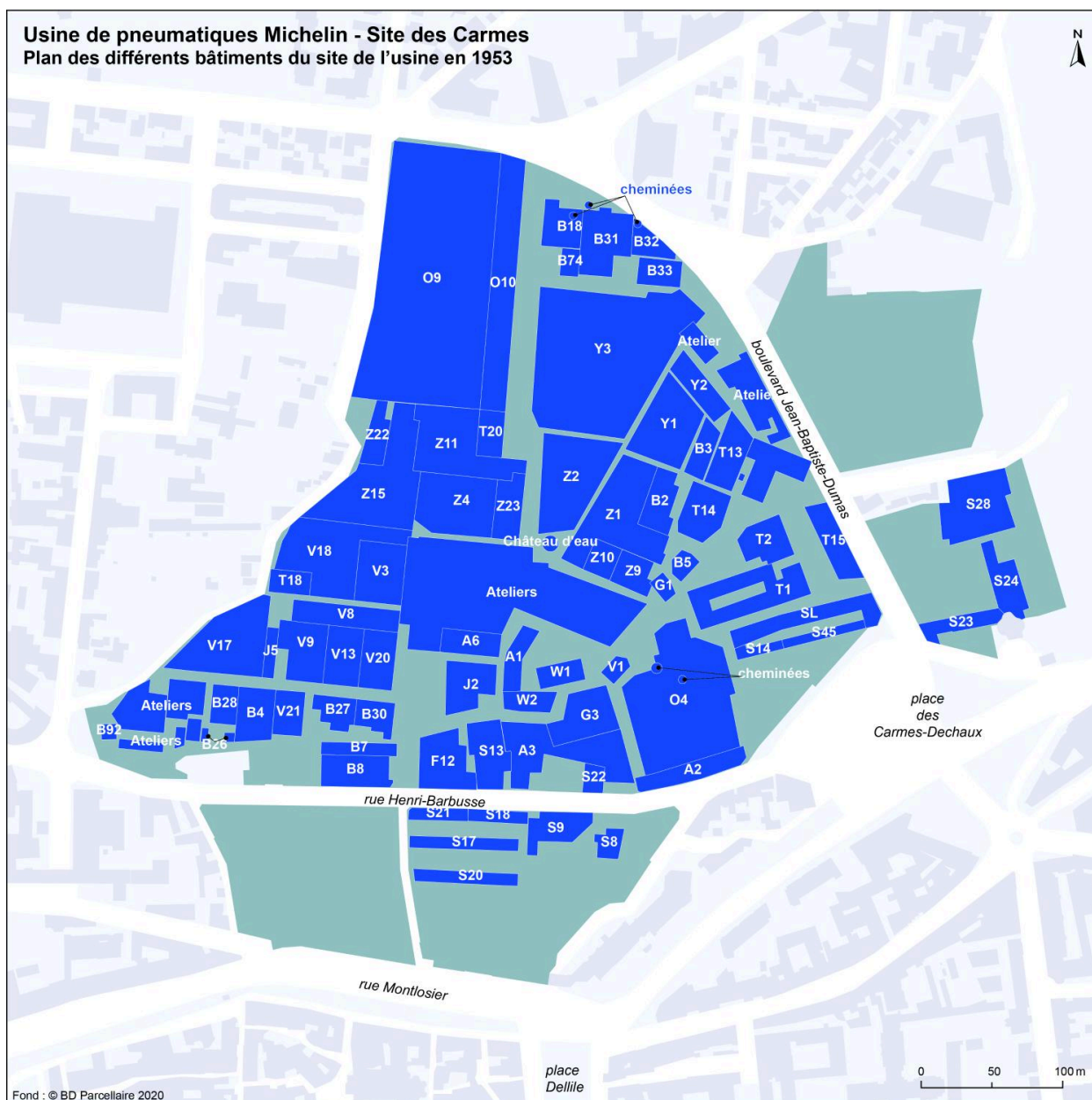
Plan numéroté des différents bâtiments du site de l'usine en 1953
