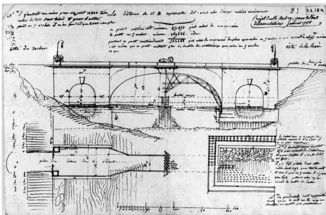
Projet de M. Aubry, pour le pont de la Mulatière, janvier 1788 / Aubry, janvier 1788
