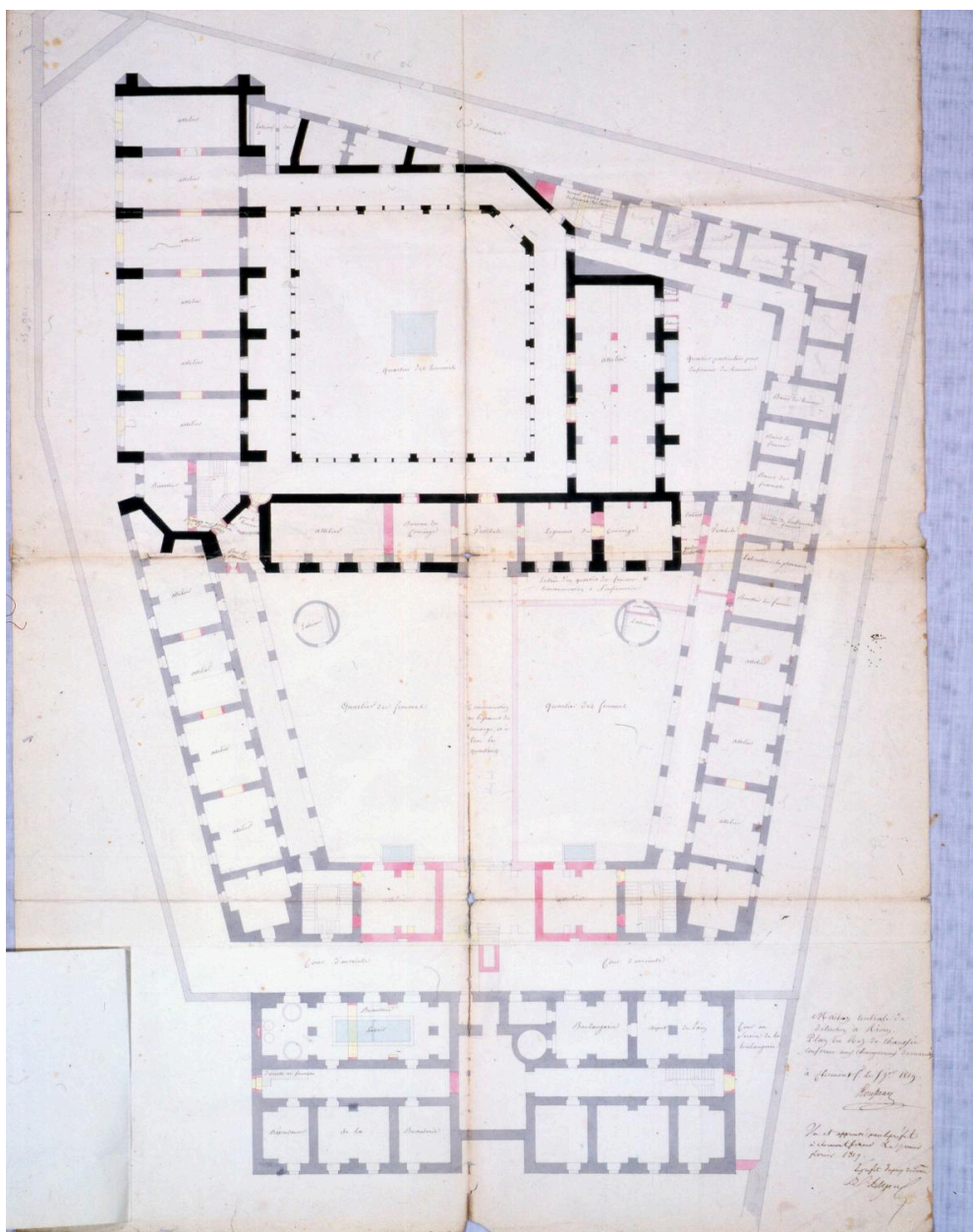
Maison centrale de détention à Riom. Plan du rez-de-chaussée (retombe relevée), lavis rose et violet, encre noire, sans échelle, 1819, par Rousseau.
