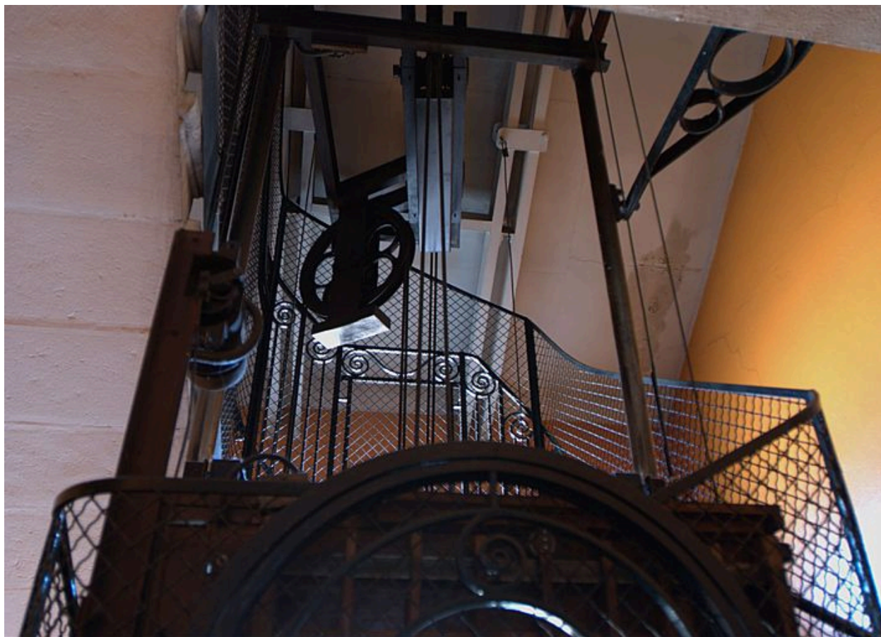
Ascenseur, détail du mécanisme
