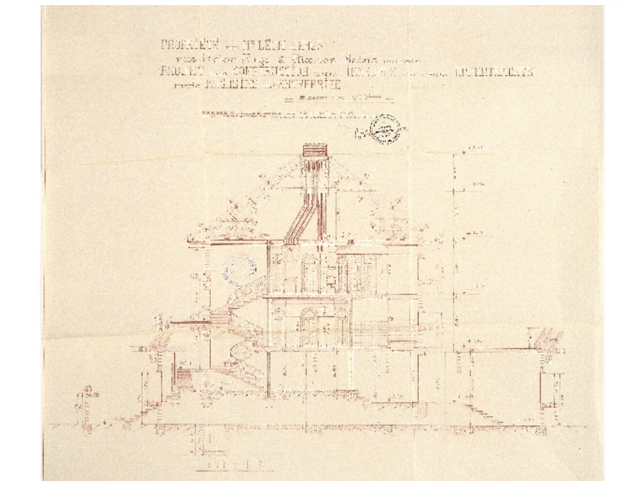
Coupe AB
