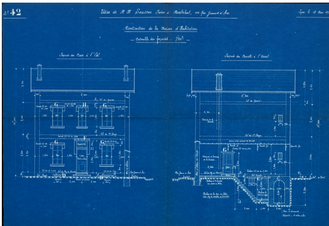
Élévation et coupe de d'une maison pour messieurs Sassac frères par M. Marvier, 1921. AC Lyon : 344 WP 093 PCA n°0158
