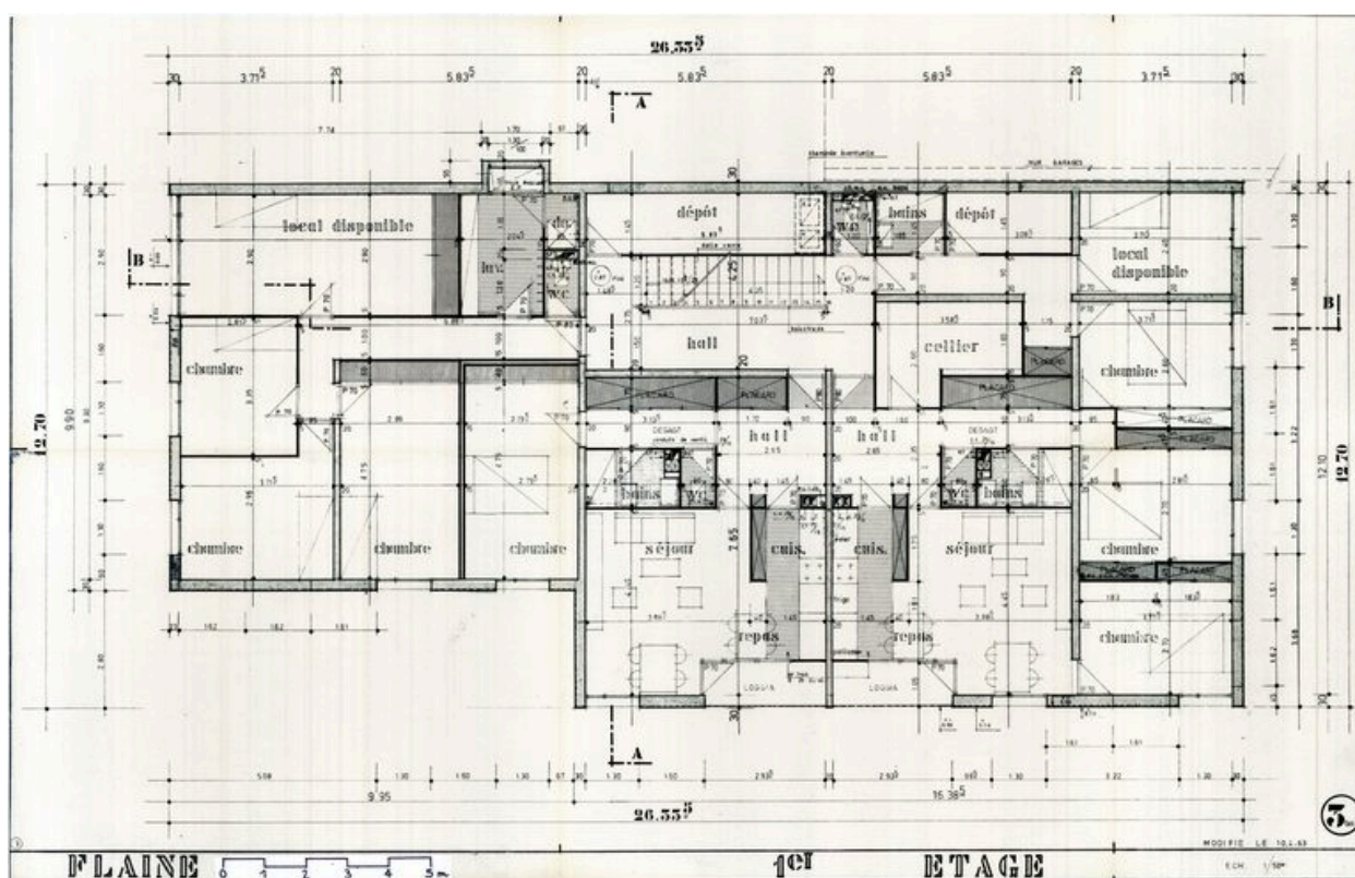
Plan du 1er étage. [Laurent Chappis, Agence Berthe, Chappis, Jomain architectes, 1962]. Modifié le 10 avril 1963 (AC Arâches-la Frasse)
