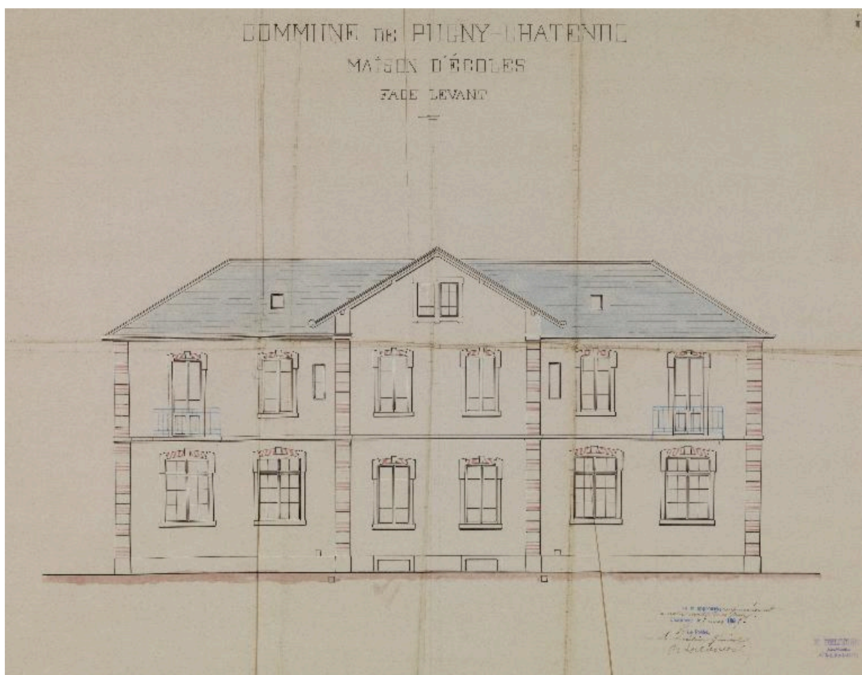
AD 73. Maison d'écoles, élévation de la façade est. 1895.
