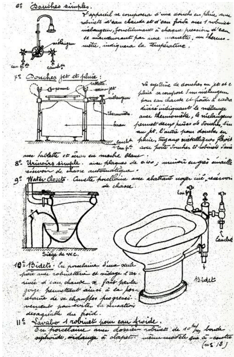
Dessin des équipements sanitaires / Tony Garnier, 30 novembre 1910
