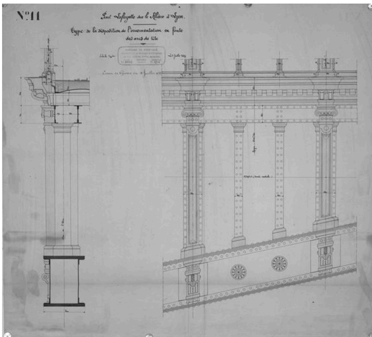
N° 11. Type de la disposition de l'ornementation en fonte des arcs de tête. 3 juillet 1889 (AD Rhône. Cie Fives-Lille. Portefeuille 368 H)
