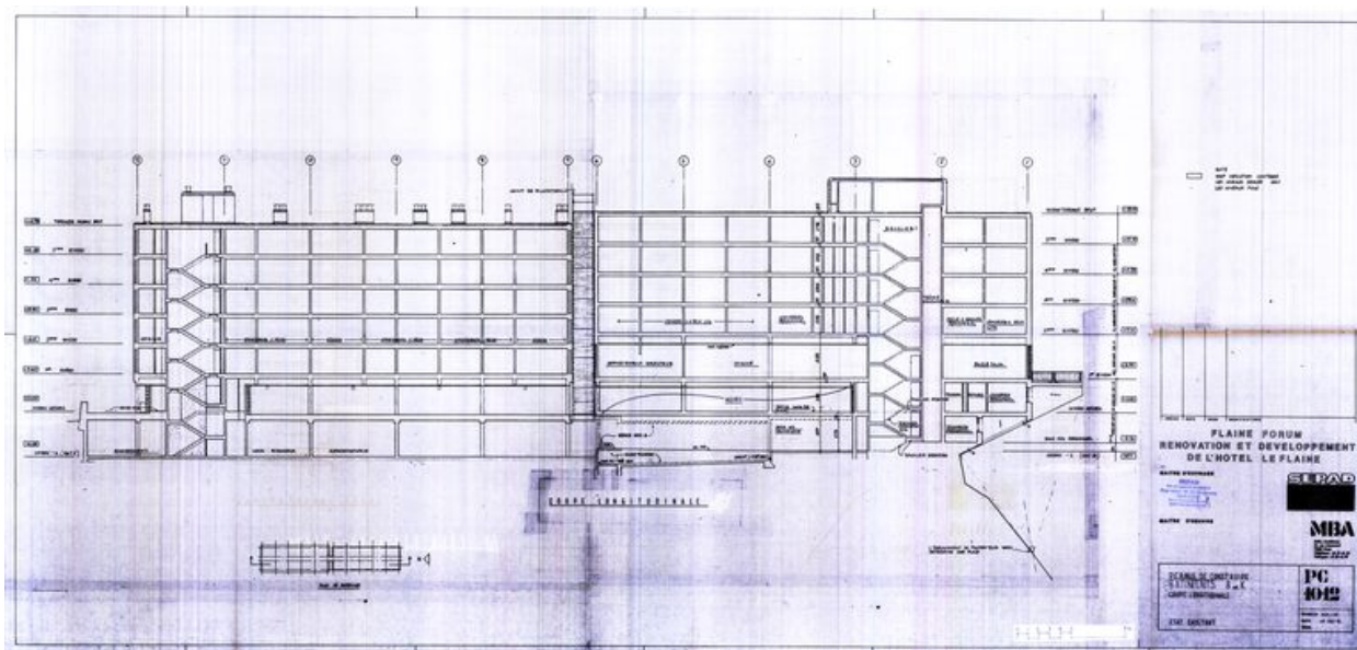
Rénovation et développement de l'hôtel le Flaine. Bâtiments B et K. Coupe longitudinale. Etat existant. MBA maître d'oeuvre, 10 mai 1991 (AC Arâches-la-Frasse)
