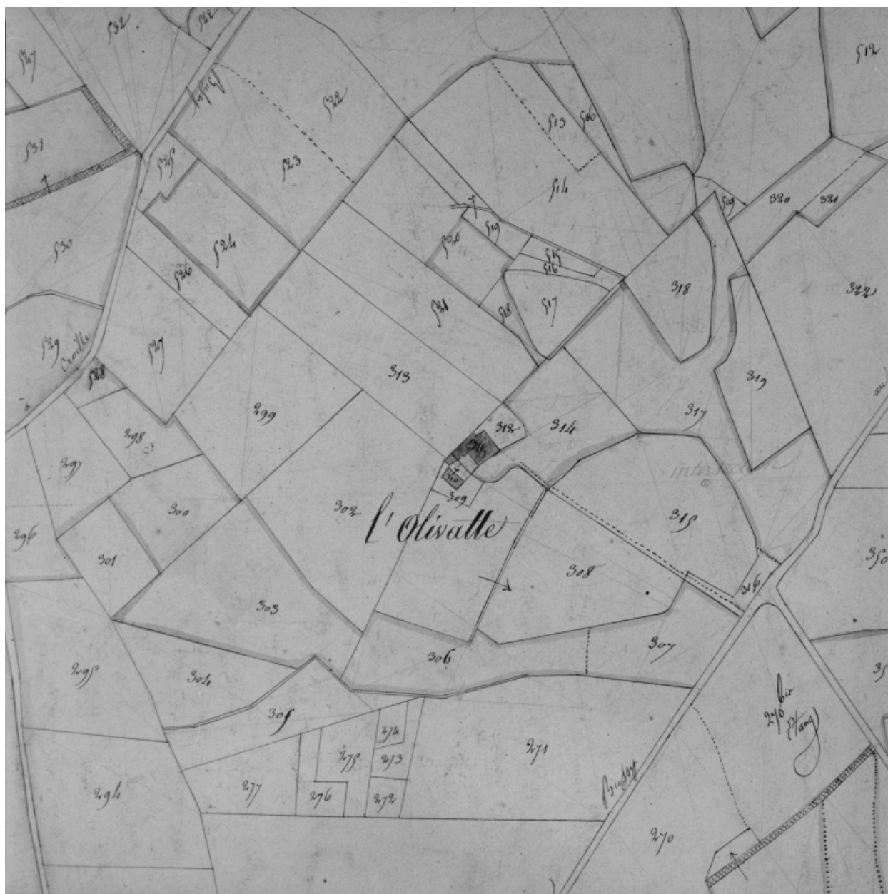
Plan cadastral ancien, 1826. Section A1, détail de l'Olivatte, échelle originale 1/2500e.
